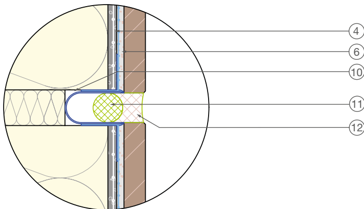
Детайл Мащаб 1:2
