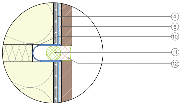
Детайл Мащаб 1:2
