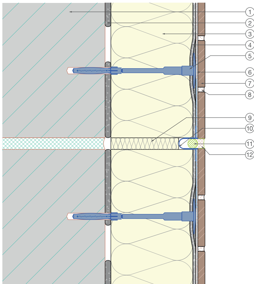
Детайл Мащаб 1:2
