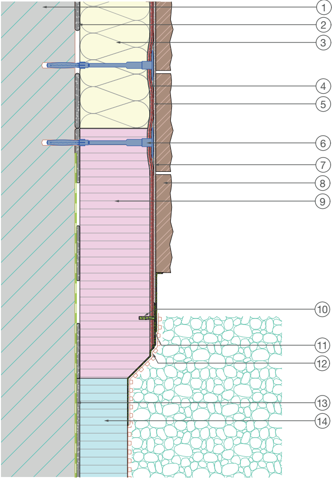
Детайл Мащаб 1:2
