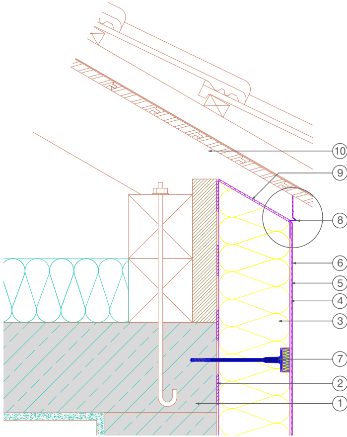
детайл мащаб 1:2
